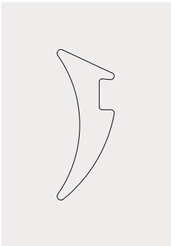
VITRA-VANDO Glas-Keilprofil EPDM-Dichtung grau VITRA-VANDO Glass wedge profile EPDM grey sealing feste Länge | fix length für 8 mm Glas | for 8 mm glass Art. 36801500135 für 10/12 mm Glas | for 10/12 mm glass Art. 36801600135 200 m für 8 mm Glas | for 8 mm glass Art. 36801500138 für 10/12 mm Glas | for 10/12 mm glass Art. 36801600138
