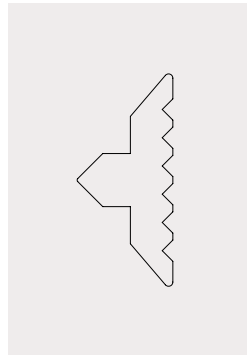
VITRA-VANDO Kontaktprofil EPDM-Dichtung grau VITRA-VANDO Contact Profile EPDM grey sealing feste Länge | fix length für 8/10/12 mm Glas | for 8/10/12 mm glass Art. 36801700135 200 m für 8/10/12 mm Glas | for 8/10/12 mm glass Art. 36801700138
